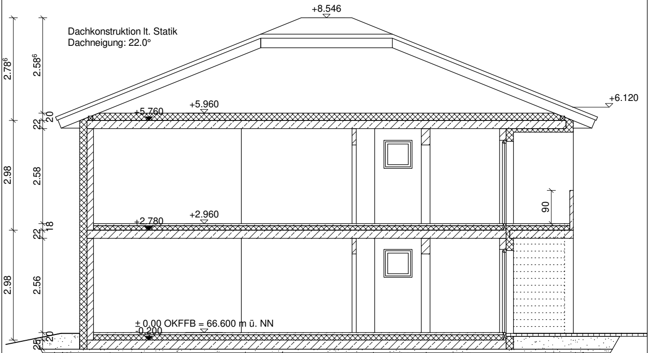
SCHNITT A-A
